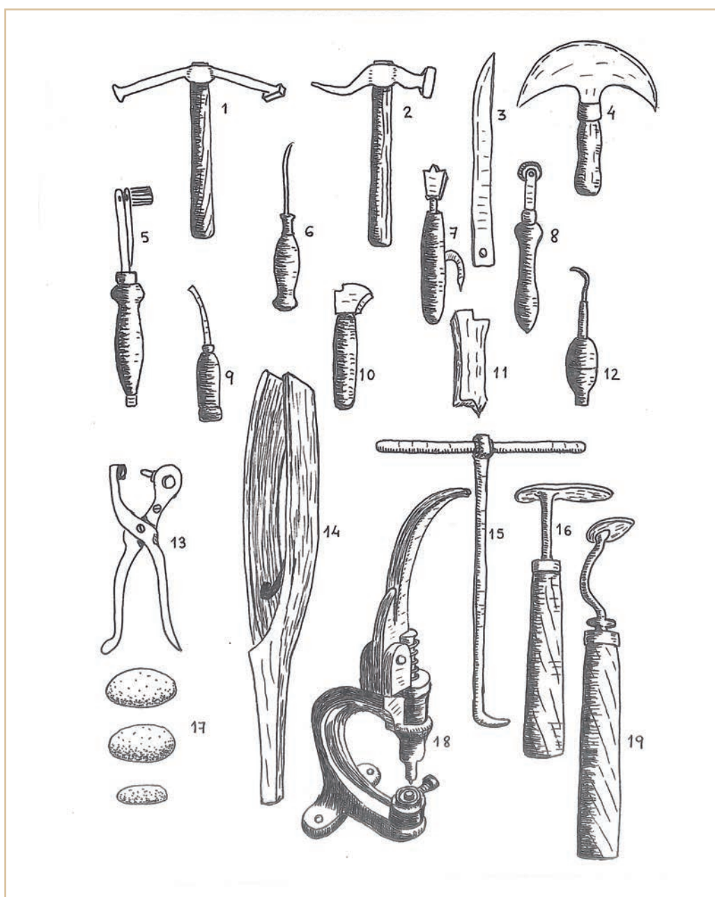
1. Martelo das solas / 2. Martelo / 3. Coitela recta / 4. Coitela curva ou media lúa / 5. Marcador das solas / 6. Subela 7. Bruñidor / 8. Ruleta / 9. Bruñidor / 10. Bruñidor / 11. Bruñidor / 12. Subela / 13. Sacabocados / 14. Prensa dos zapatos 15. Tiraformas / 16. Bigornia recta / 17. Coios / 18. Bigornia recta / 19. Bigornia curva.
