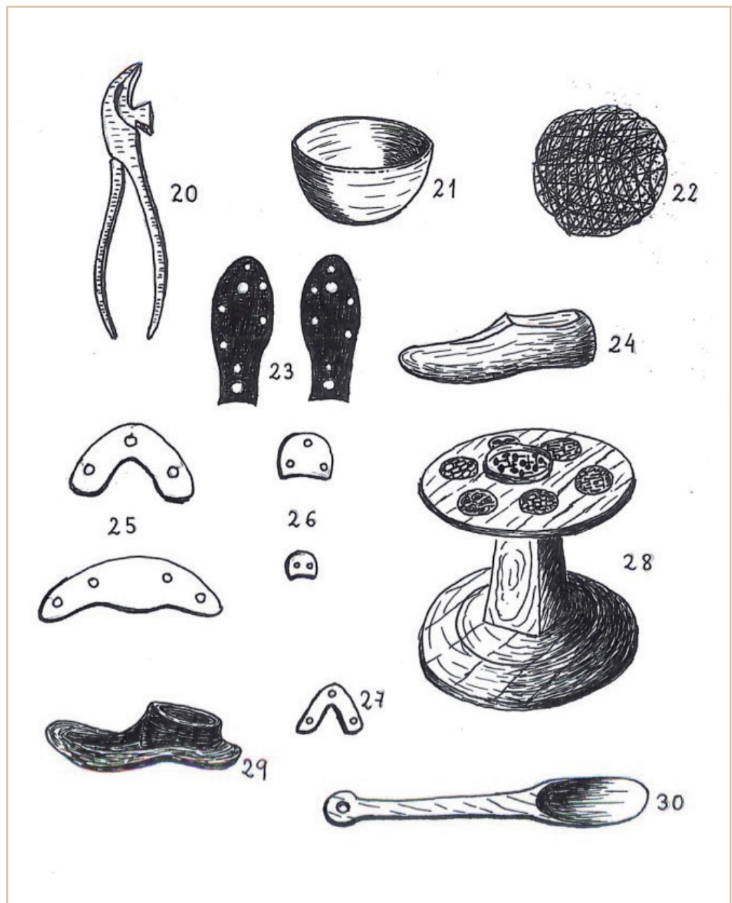
20. Tenaces das tiras / 21. Cunha do pez / 22. Pez / 23. Formas das solas / 24. Forma dos zapatos / 25. Defensas / 26. Tapas / 27. Punteira / 28. Mesa xiratoria / 29. Forma de ferro / 30. Calzador.
